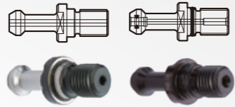
Type C 拉桿 Pull Stud
